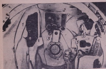
Дитынэ жь һөндөр'ө кабинэ космоседе гоми—торэри'а «Восток»-те: 1—шутла фэр'эчэч; 2—г'эхе һаттына г'эубэуэсэ; 3—камера лурдэуэлтэ- лэ; 4—дидиматор һаттына оптикэсэ; 5—дэстне сэр'гарырына гомийи ориентэсэ; 6—р'адийо-дидэч; 7—контэйнера ште х'эбэч;
