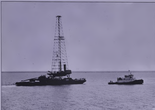
برج الحفر أثناء قطره عبر خور الصبية الى بوبيان
